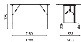
Rico Table Plateau 120 x 80
