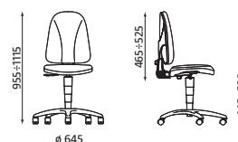
Mécanisme CPT largeur d'assise : 460 profondeur d'assise : 450
