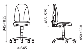
Mécanisme ACTIVE 1 largeur d'assise : 460 profondeur d'assise : 450
